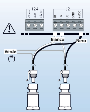
4-20 mA Probe:
